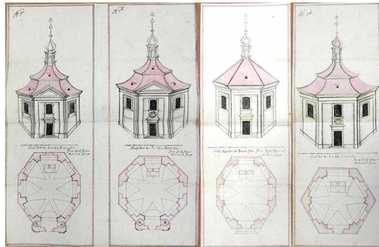
Obr. 1 Pavel Ignác Bayer, návrhy votivní (děkované) kaple Nejsvětější Trojice morových patronů v Libniči, leden 1714 (pozn. zvítězil 3. návrh)
